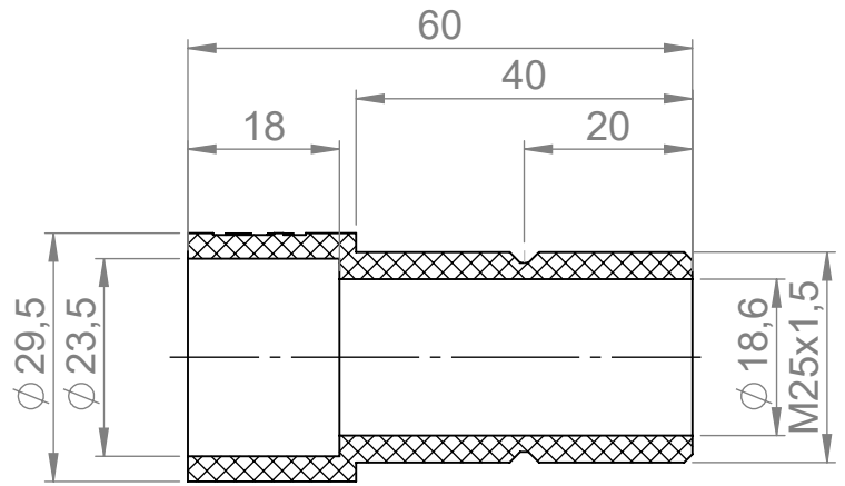
SCHNITT A-A
