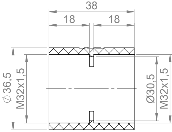
SCHNITT A-A
